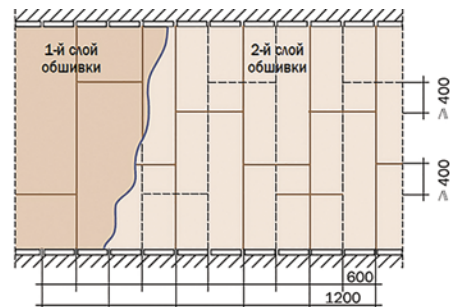
Рис. 14. Схема обшивки листами ГКЛ
