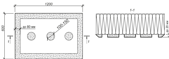
Рис. 28. Схема нанесения клея контурно-маячковым способом
