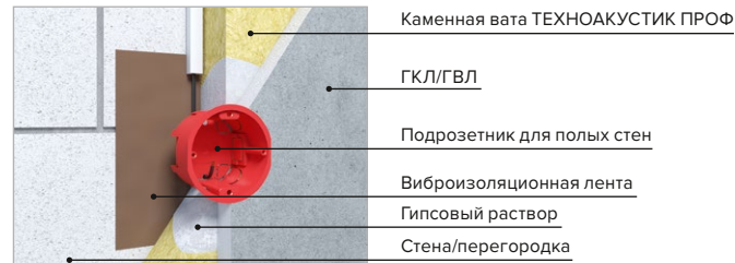
Рис. 18 б. Вариант монтажа электропроводки в кабель-каналах и подрозетника с монтажом в гипсовую смесь
