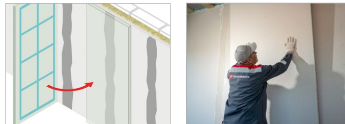
Рис. 15. Крепление листов ГКЛ/ГВЛ второго слоя
