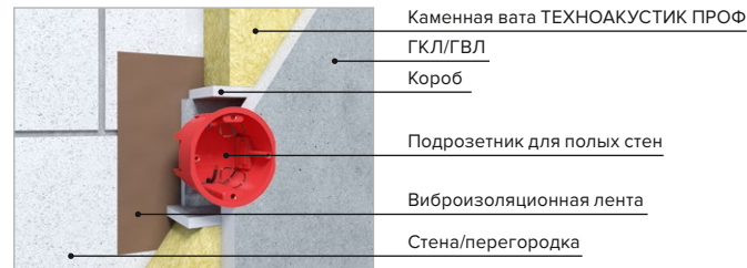
Рис. 18 в. Вариант монтажа электропроводки в несущей стене и подрозетника с монтажом в специальный короб
